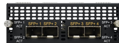
4x SFP+ Module (EXM-4F)
